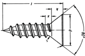
UNI 6955 DIN 7982 TESTA CILINDRICA PAN HEAD
