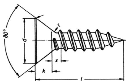
TESTA PIANA SVASATA
