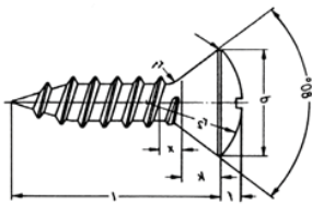
UNI 6956 DIN 7983
