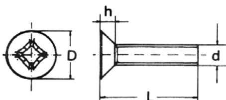
UNI 7688 DIN 965 TESTA PIANA SVASATA FLAT HEAD
