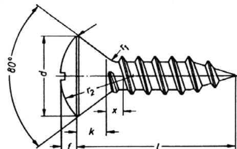
TESTA SVASATA CALOTTA
