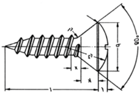
UNI 6956 DIN 7983 TESTA GOCCIA SEGO OVAL FLAT HEAD
