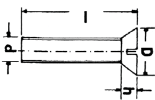
UNI 6109 DIN 963
