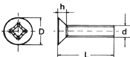
UNI 7688 DIN 965 TESTA PIANA SVASATA FLAT HEAD
