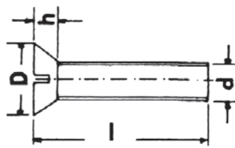
UNI 6109 DIN 963 TESTA PIANA SVASATA FLAT HEAD
