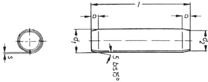
SIGLA SESX esempio SESX 4X20 GR
