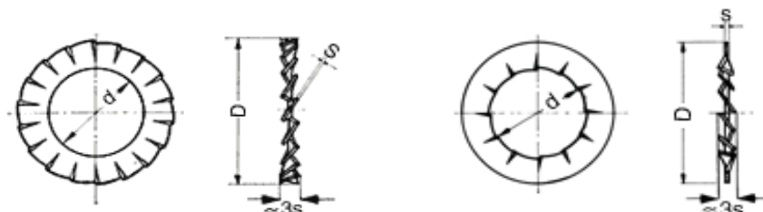
DIN 6798/A DENTELLATA ESTERNA
