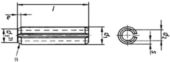
SIGLA SEPX esempio SEPX 4X20 GR
