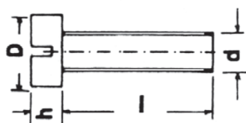
UNI 6107 DIN 84 TESTA CILINDRICA PAN HEAD
