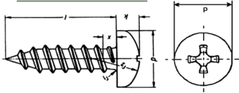
UNI 6954 DIN 7981
