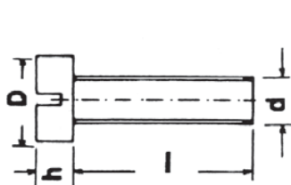
UNI 6107 DIN 84 TESTA CILINDRICA PAN HEAD
