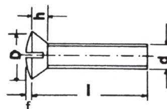
UNI 6110 DIN 964 TESTA GOCCIA SEGO OVAL FLAT HEAD
