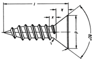
UNI 6955 DIN 7982
