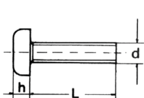
UNI 7687 DIN 7985 TESTA CILINDRICA PAN HEAD
