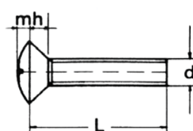
UNI 7689 DIN 966 TESTA GOCCIA SEGO OVAL FLAT HEAD
