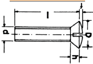
UNI 6110 DIN 964 TESTA GOCCIA SEGO OVAL FLAT HEAD
